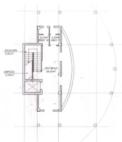
ALTERNATIVA Nº4 PLANTA BAJA ESCALA: 1/100
