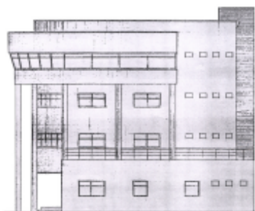
ALZADO LATERAL
